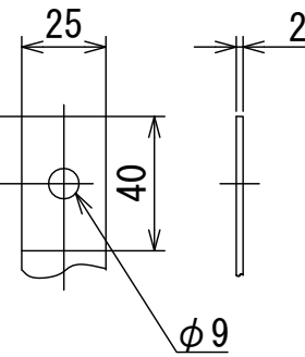
一次端子詳細図
