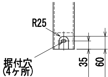
据付部上面図
