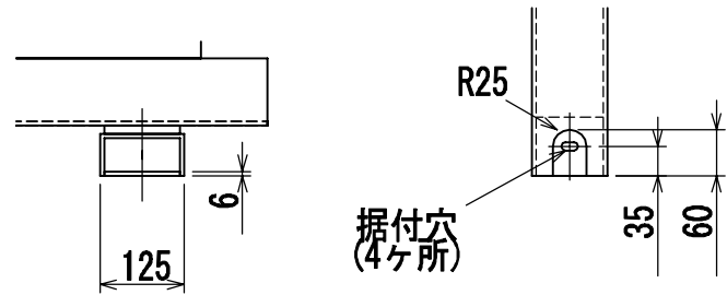
据付部正面図
