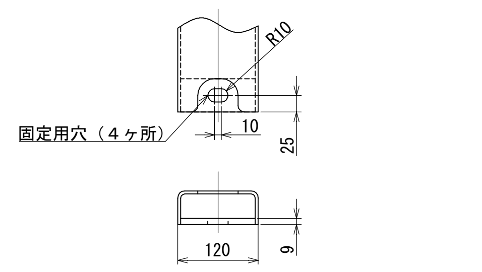
固定部詳細図
