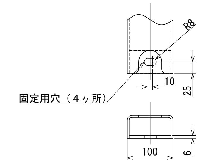
固定部詳細図
