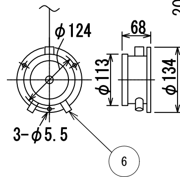
一次端子詳細図
