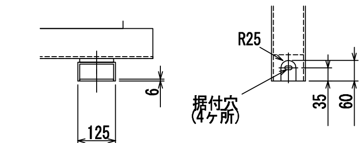
据付部正面図
