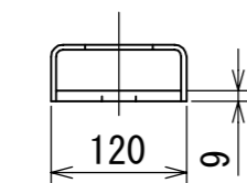
固定部詳細図
