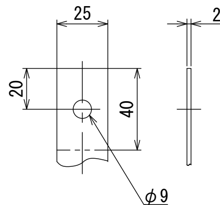
一次端子詳細図
