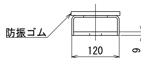
固定部詳細図
