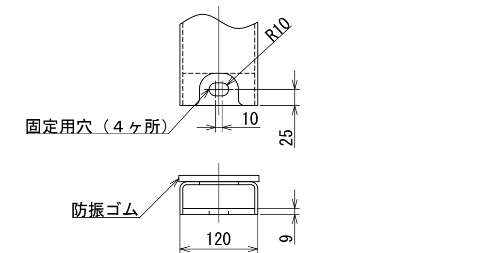
固定部詳細図
