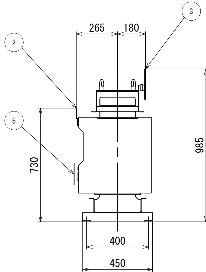
一次端子詳細図
