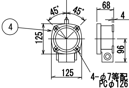
一次端子詳細図
