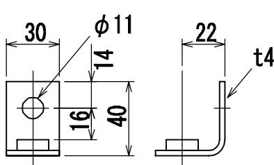
二次端子詳細図
