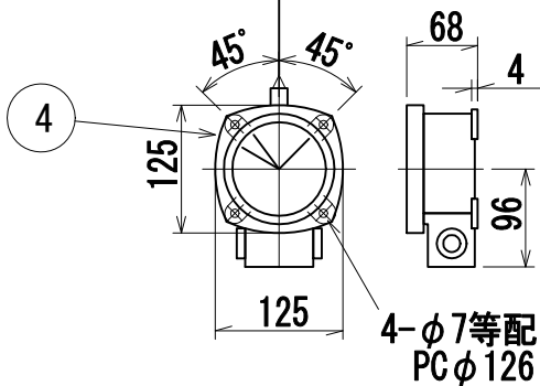
一次端子詳細図
