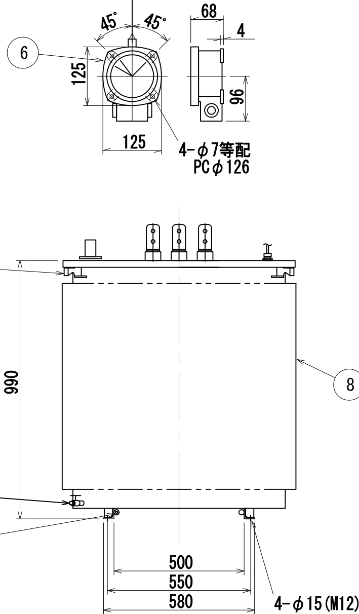
一次端子詳細図
