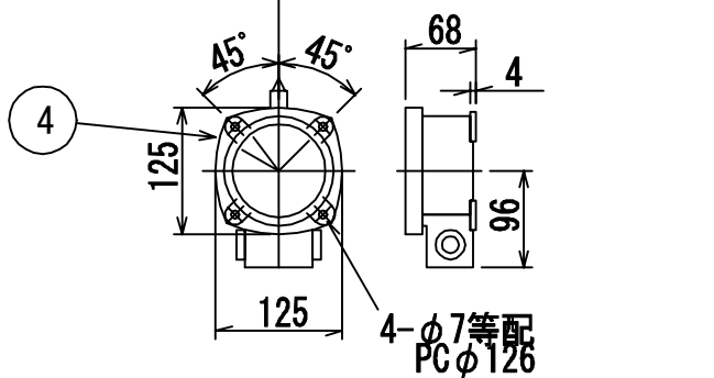
一次端子詳細図
