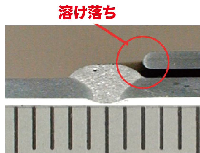
レーザ溶接
