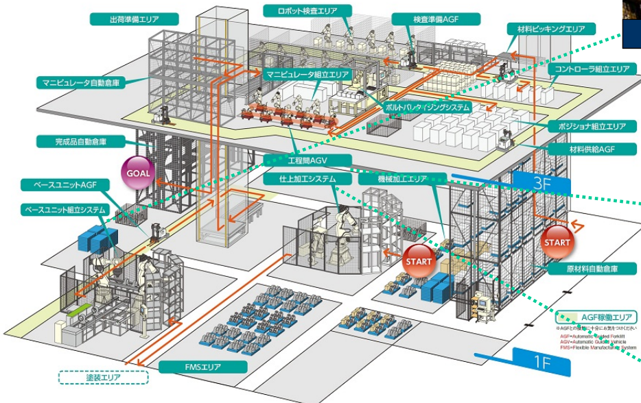
ベースユニット組立システム
